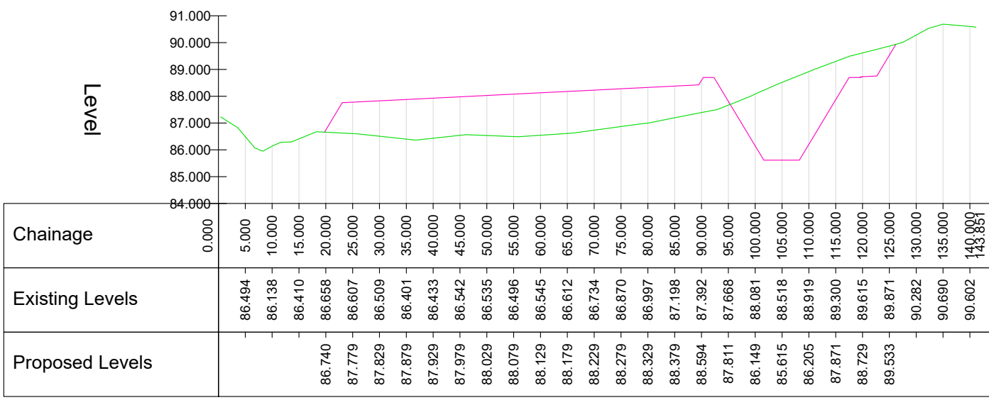
X-SECTION 10 - LONGSECTION SCALE: H 1:1000,V 1:200. DATUM: 84.000
