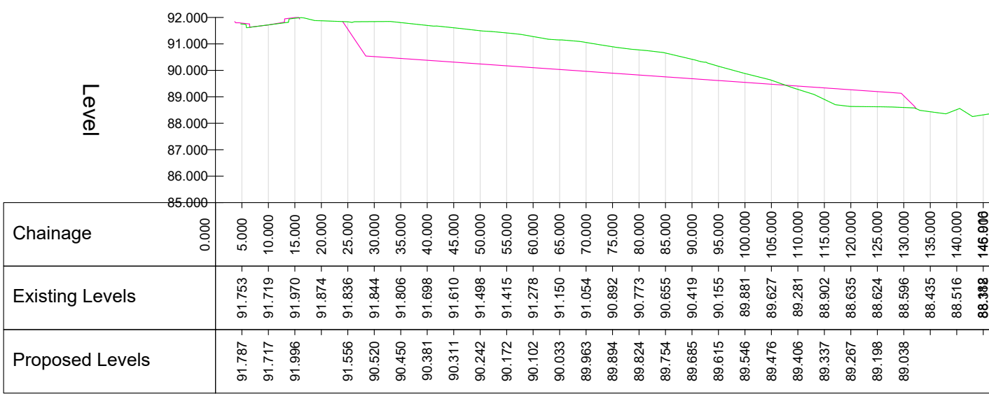
X-SECTION 2 - LONGSECTION SCALE: H 1:1000,V 1:200. DATUM: 85.000
