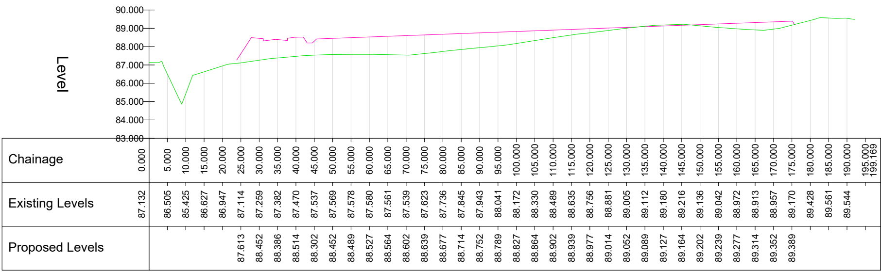
X-SECTION 8 - LONGSECTION SCALE: H 1:1000,V 1:200. DATUM: 83.000
