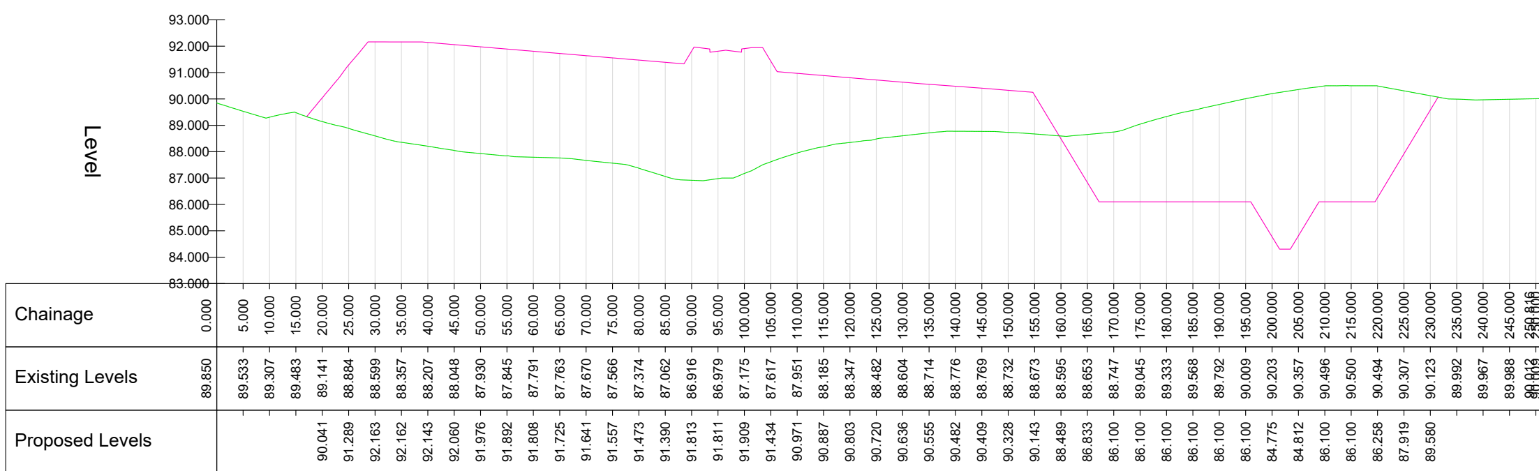
X-SECTION 5 - LONGSECTION SCALE: H 1:1000,V 1:200. DATUM: 83.000
