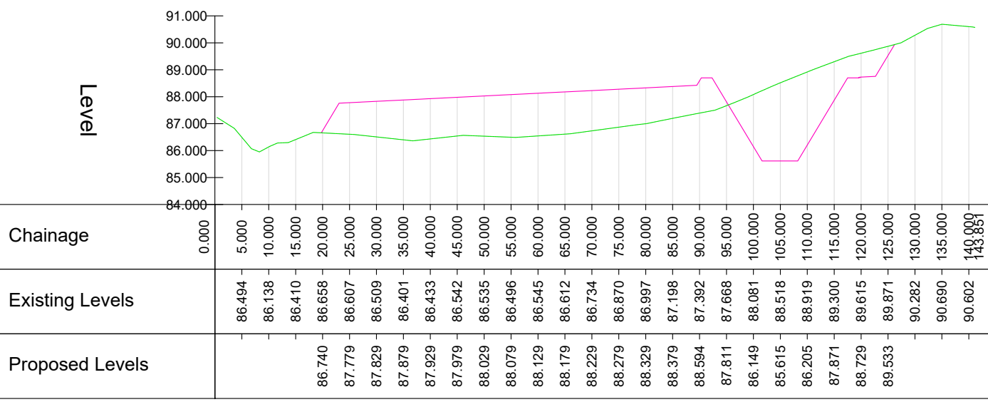
X-SECTION 10 - LONGSECTION SCALE: H 1:1000,V 1:200. DATUM: 84.000
