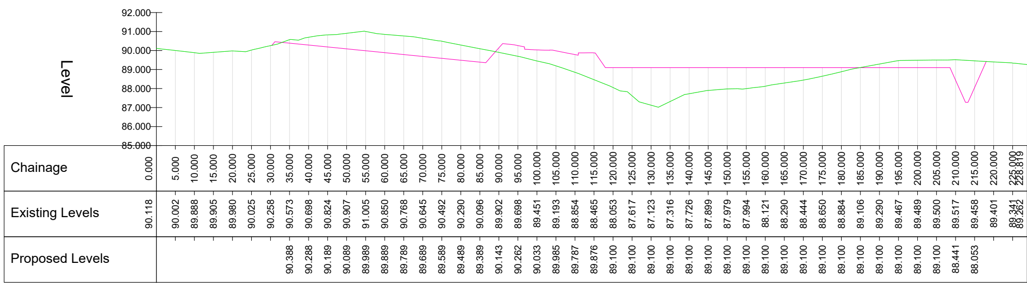
X-SECTION 1 - LONGSECTION SCALE: H 1:1000,V 1:200. DATUM: 85.000
