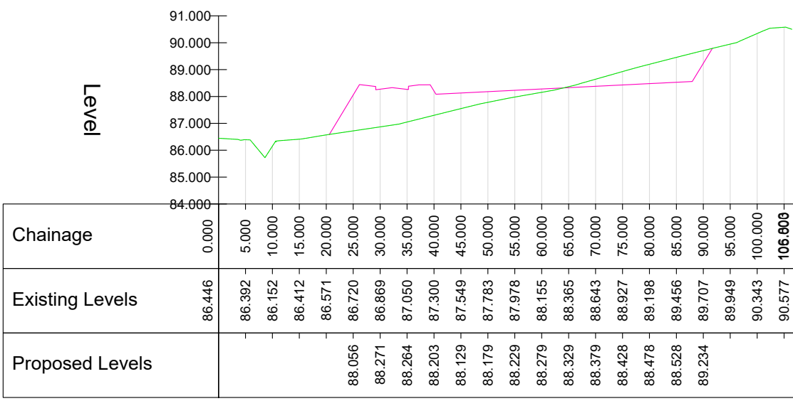
X-SECTION 9 - LONGSECTION SCALE: H 1:1000,V 1:200. DATUM: 84.000
