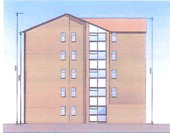
② Elevation 2 - a 1 : 100
